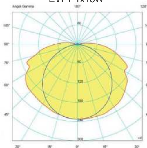
EVFT 1x18W
