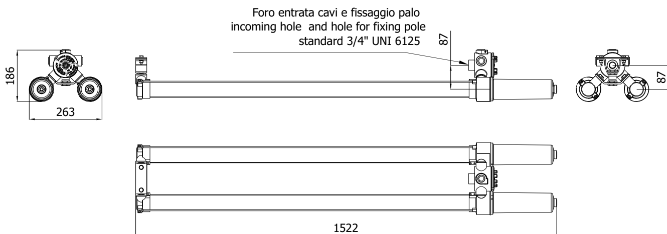
Fissaggio su palo lampada doppia Double lamp pole mounting
