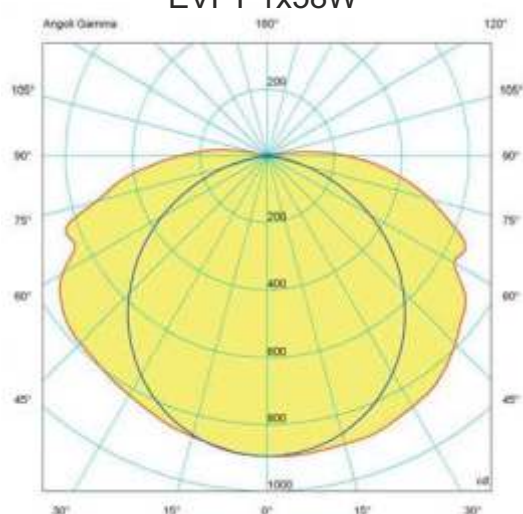
EVFT 1x58W
