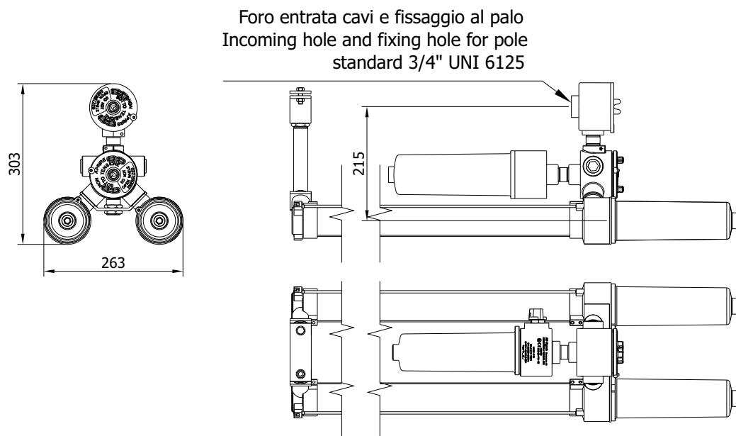
Fissaggio su palo lampada doppia con emergenza Double lamp pole mounting with emergency
