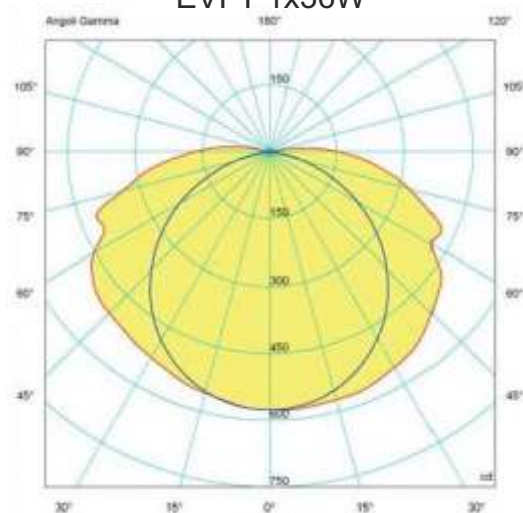
EVFT 1x36W
