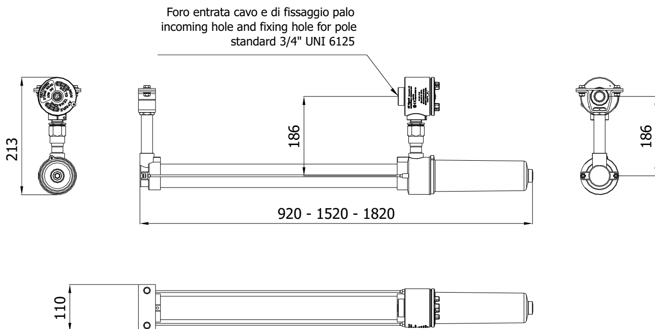
Fissaggio su palo lampada singola Single lamp pole mounting
