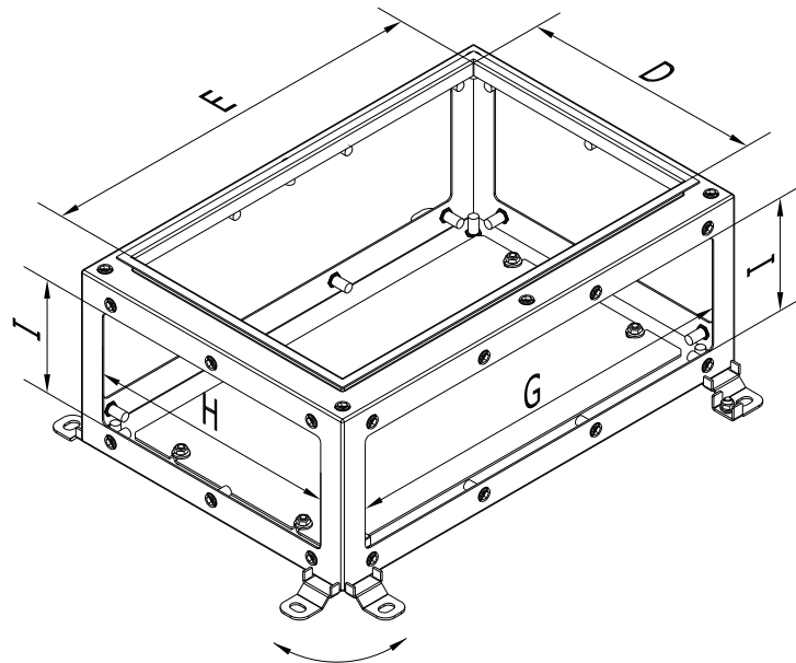
VITE DI TERRA M6 EARTH SCREW M6
