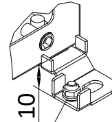
VITE DI TERRA M6 EARTH SCREW M6
